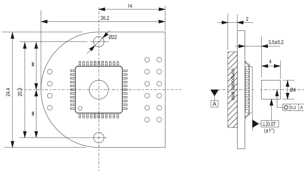
Fig. 37: RMK3B dimensions
