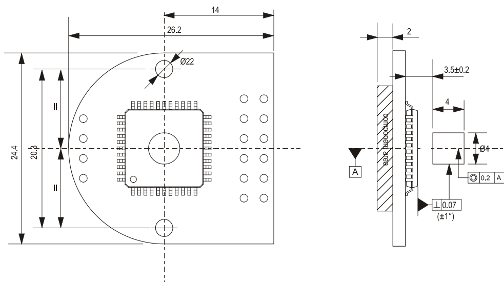
Fig. 37: RMK3B dimensions
