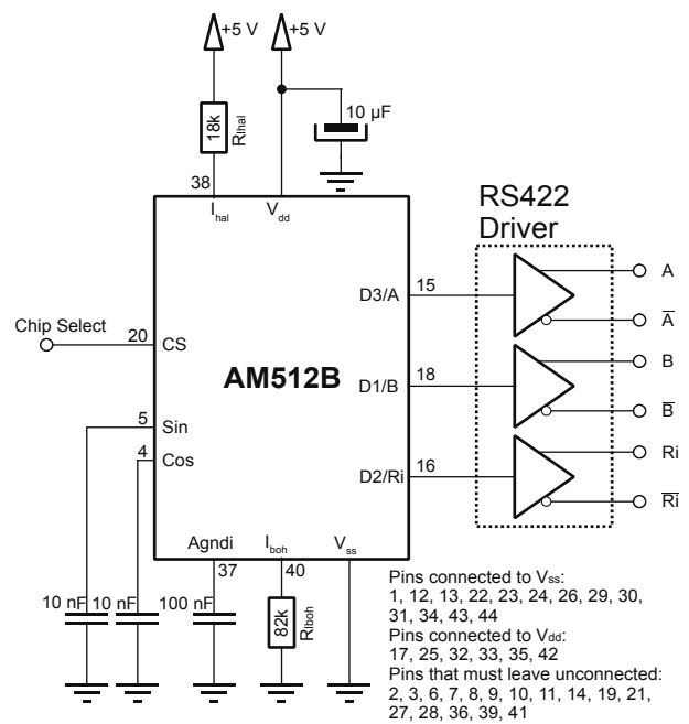
Fig. 28: Incremental output
