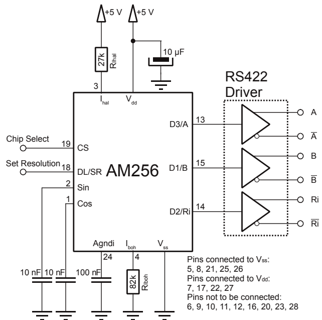
Fig. 21: Incremental output
